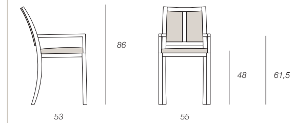
Poltroncina con seduta imbottita Wooden armchair with upholstered seat Armstuhl mit gepolstertem Sitz
